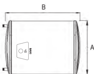
Instalación Horizontal
