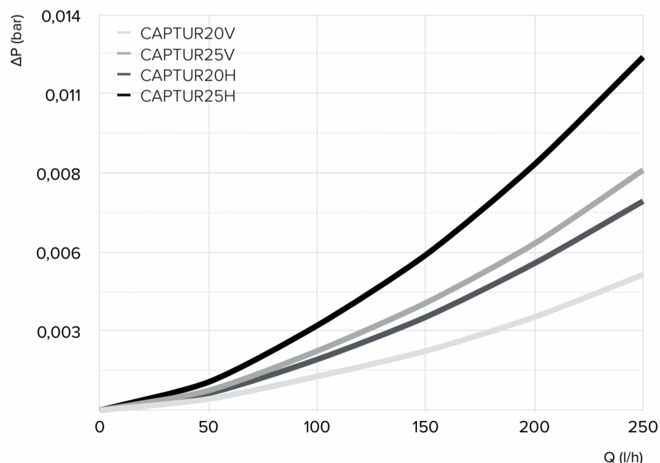
Pérdida de carga en captadores GH-CAPTUR
